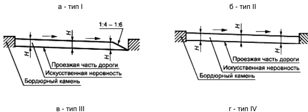
Рисунок 2 - Продольные профили ИН
